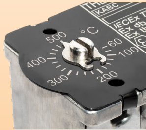
C: 螺丝刀的型号，带箭头和印刷的铝表盘，用于 JPCI 或其他供应商的 PPS Ex-c 外壳进行伴热；
