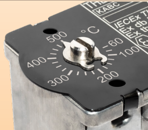
C: 螺丝刀的型号，带箭头和印刷的铝表盘，用于 JPCI 或其他供应商的 PPS Ex-c 外壳进行伴热；
